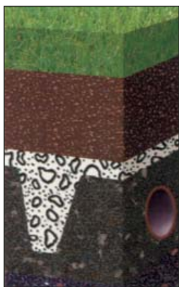
Schichtaufbau einer KRESCAT-Rasenfläche nach DIN 18035, Teil 4: Bodennahe Bauweise
