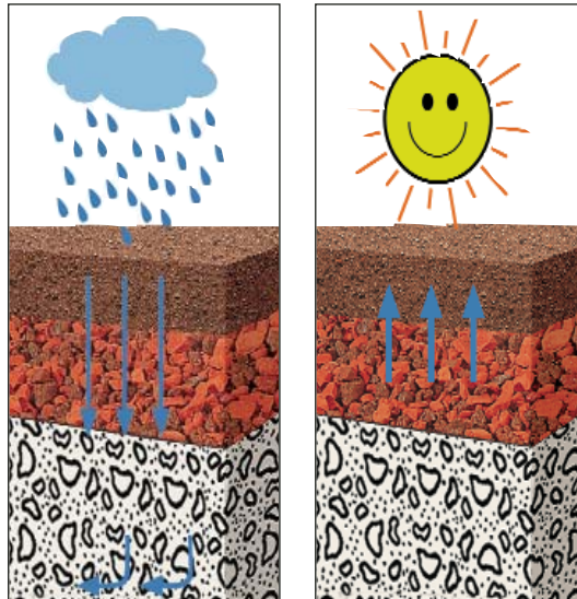
Schichtaufbau BERGOLIT
